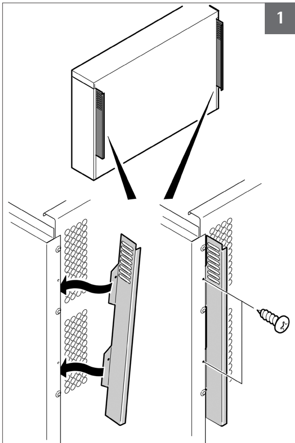
Abbildung 1: Die beiliegenden, seitlichen Wandabstandsleisten werden zwischen Rückwand und Seitenteil geschoben und anschliessend mit den beiliegenden Schrauben verschraubt (siehe 4.2.1). Bei Geräteserie Flach sind die Leisten bereits montiert.
